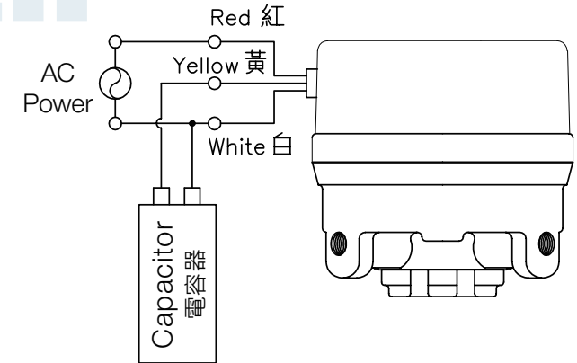
Wiring 電容器配線圖
