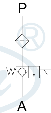
Diagram 油路圖
