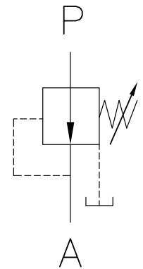
Diagram 油路圖
