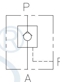
Diagram 油路圖
