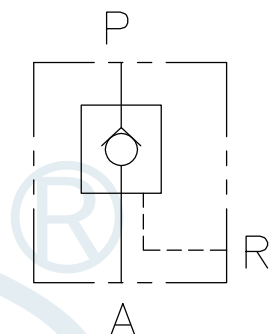
Diagram 油路圖
