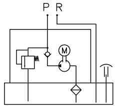
Diagram 油路圖
