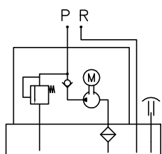
Diagram 油路圖
