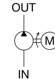
Diagram 油路圖
