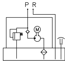
Diagram 油路圖
