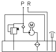
Diagram 油路圖
